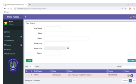
Gambar 7 Menu Terapis
