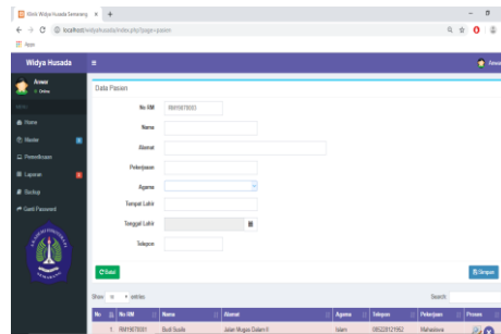
Gambar 6 Menu Pasien
