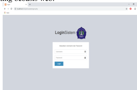
Gambar 10 Halaman Login
