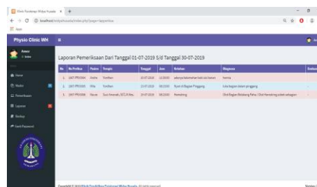
Gambar 9 Laporan Pemeriksaan
