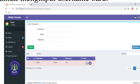
Gambar 8 Menu Admin
