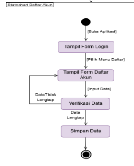
Gambar 6. Statechart Diagram Daftar Akun
