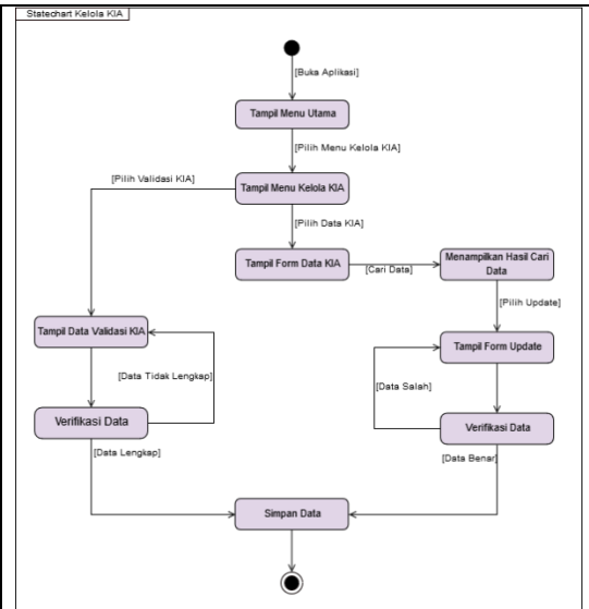
Gambar 5. Statechart Diagram Kelola KIA
