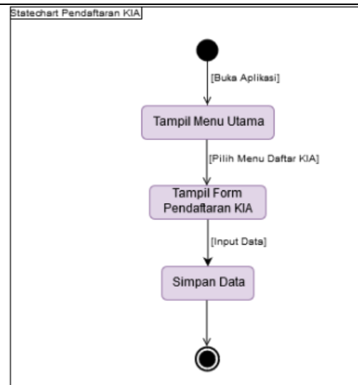
Gambar 7. Statechart Diagram Pendaftaran KIA
