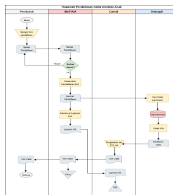
Gambar 2. Flowchart Sistem yang Berjalan
