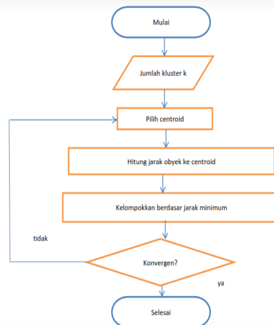
Gambar 2 Langkah proses clustering dengan k-means
