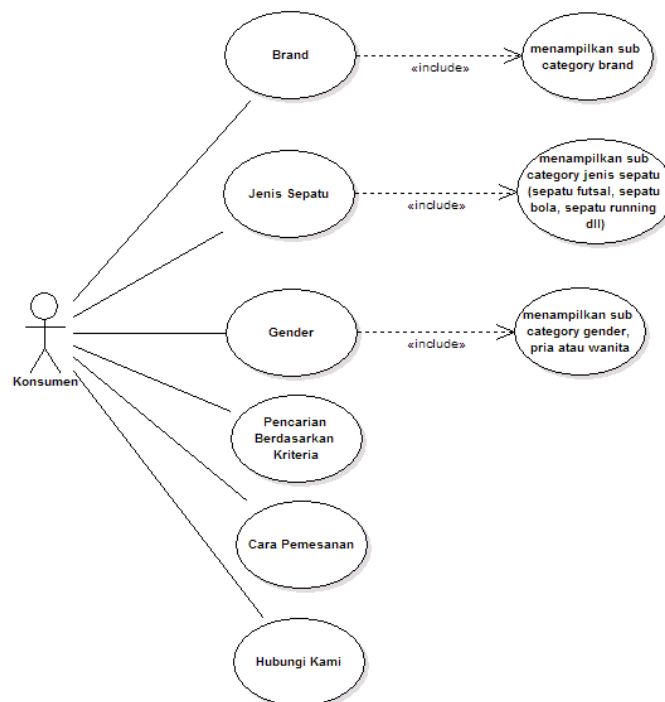
Gambar 1 : Diagram use case aplikasi pemilihan sepatu
