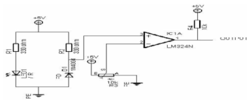
Gambar 2.5 Rangkaian sensor garis menggunakan IC LM 324
