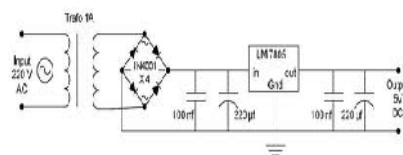
Gambar 5.5 Rangkaiann Catu daya
