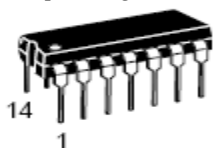
Gambar 2.4 IC LM 324 (Data sheet LM324)
