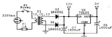
Gambar 10 Rangkaian Catudaya
