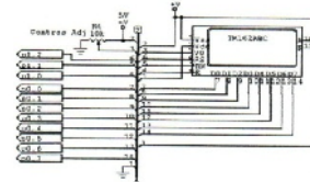
Gambar 7 Rangkaian Koneksi Display LCD
