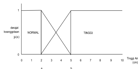
Gambar 1. fungsi keanggotaan sensor 1 maupun sensor 2
