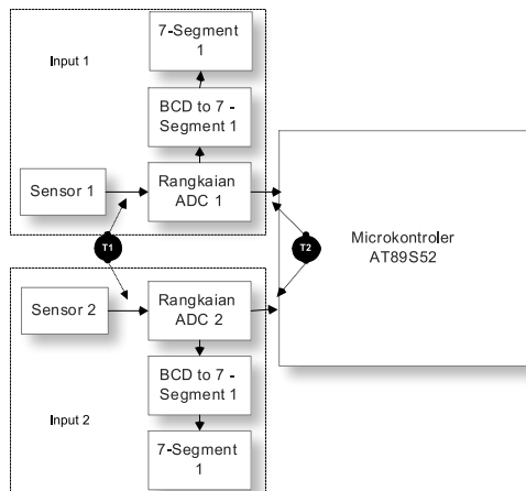
Gambar 5. Blok Pengukuran untuk Input dari sensor 1 dan 2
