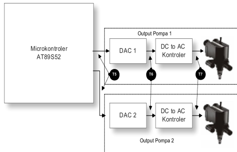
Gambar 6. Blok Pengukuran untuk output ke pompa 1 dan 2
