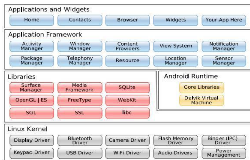
Gambar 3. Arsitektur Android
