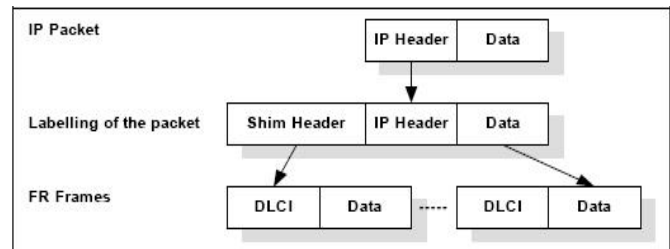
Gambar 6. Frame Relay sebagai layer Data Link
