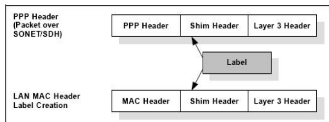
Gambar 7. Shim Header MPLS antar layer 2 dan layer 3
