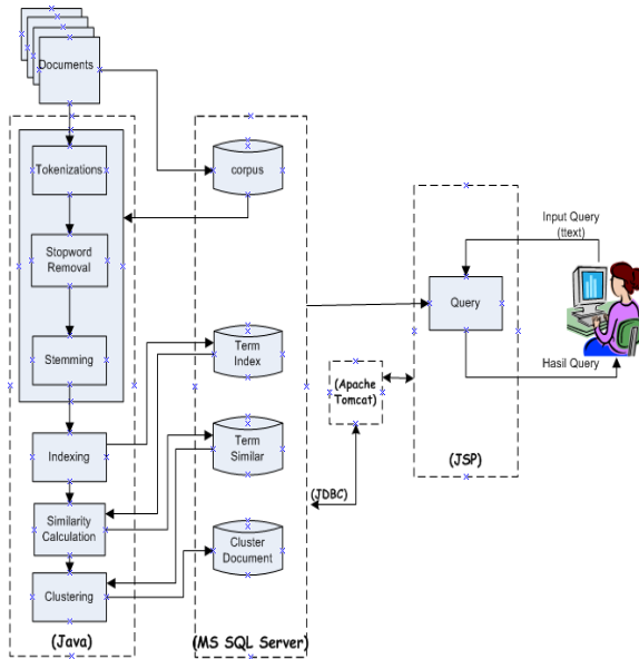
Gambar 6. Implementasi Arsitektur Sistem Temu Kembali Informasi
