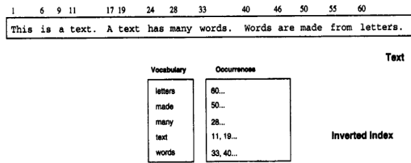
Gambar 1 Contoh Teks dan Inverted File -nya
