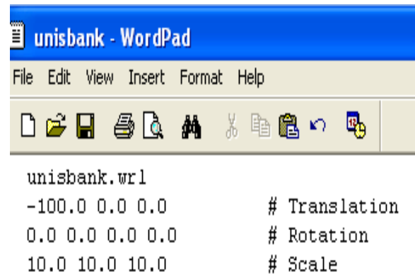
Gambar 11.b. Seting pada file unisbank.DAT
