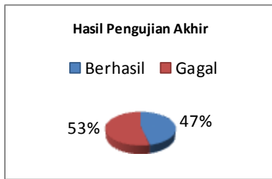
Gambar 7. Prosentase pengujian
