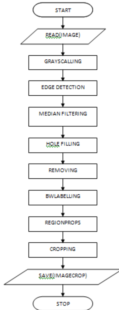
Gambar 3. Alur Algoritma
